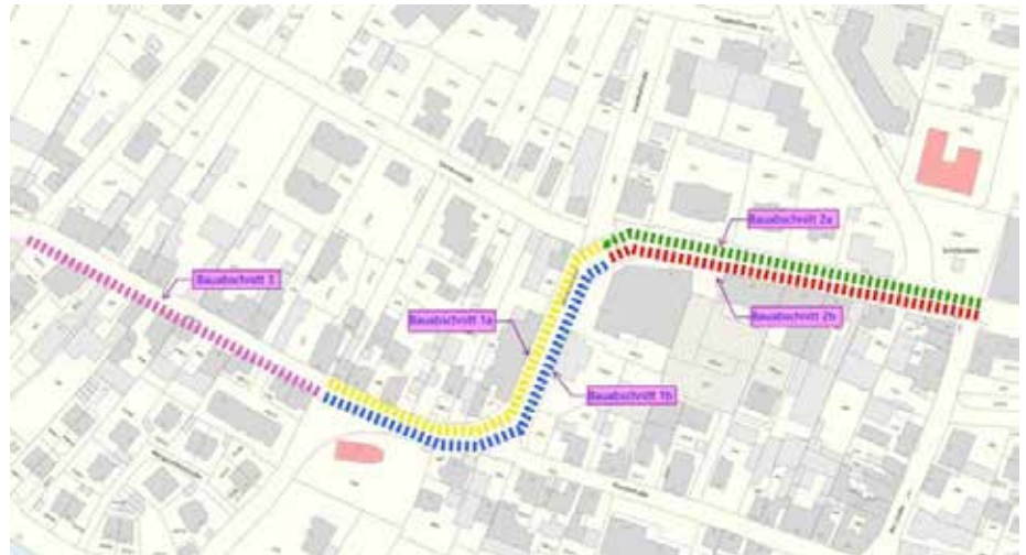
Bauabschnittplan (Quelle: Stadtwerke MüllheimStaufen GmbH)
