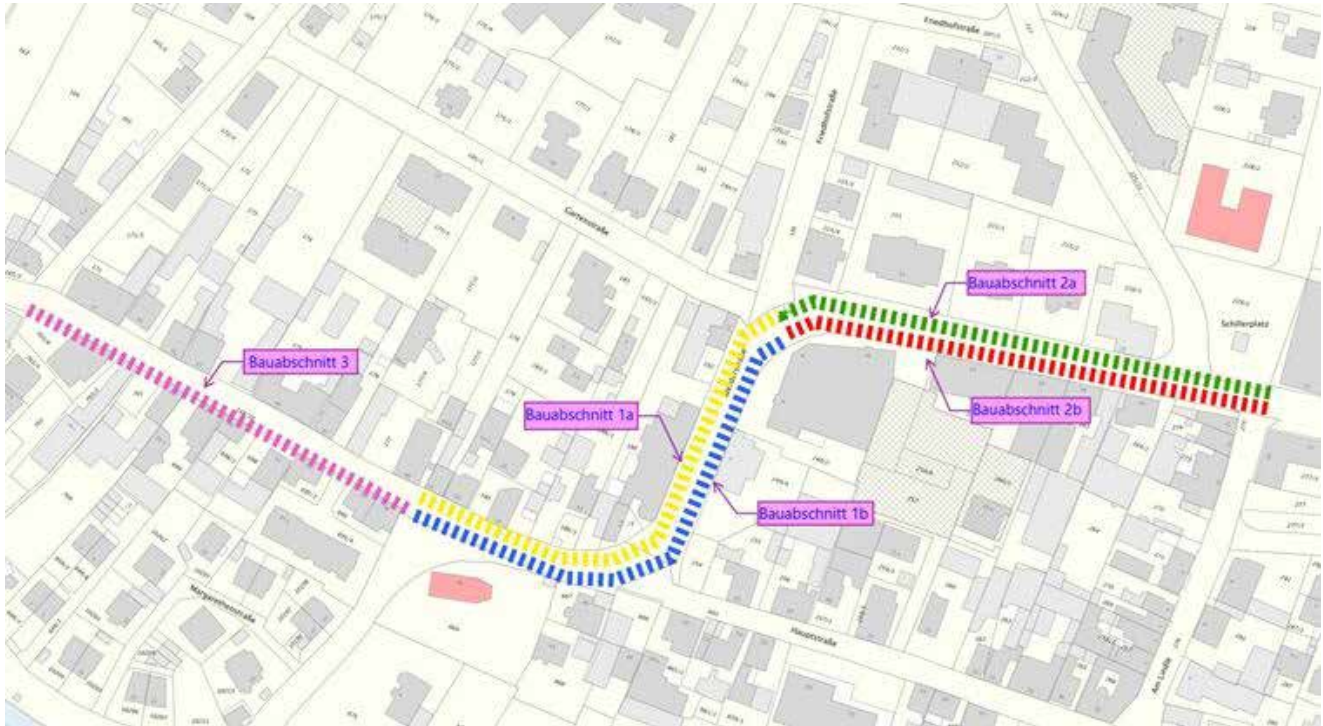
Bauabschnittplan (Quelle: Stadtwerke MüllheimStaufen GmbH)
